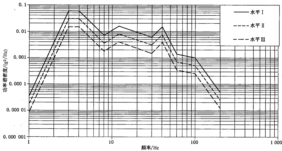
图 A.1 公路运输不同严酷水平随机振动 PSD 曲线
